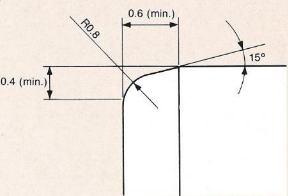
Fig. 8 Shaft chamfer
